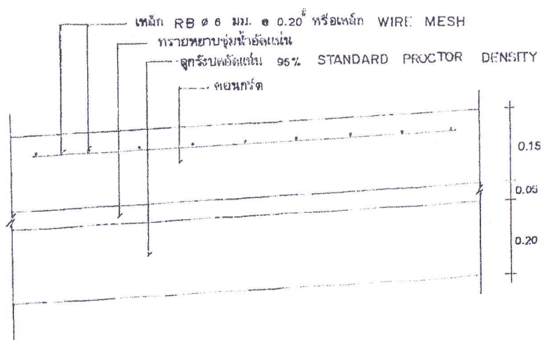
รายละเอียดขนาดคอนกรีตเสริมเหล็ก
